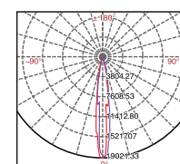
NLED1151N 30W 15°
